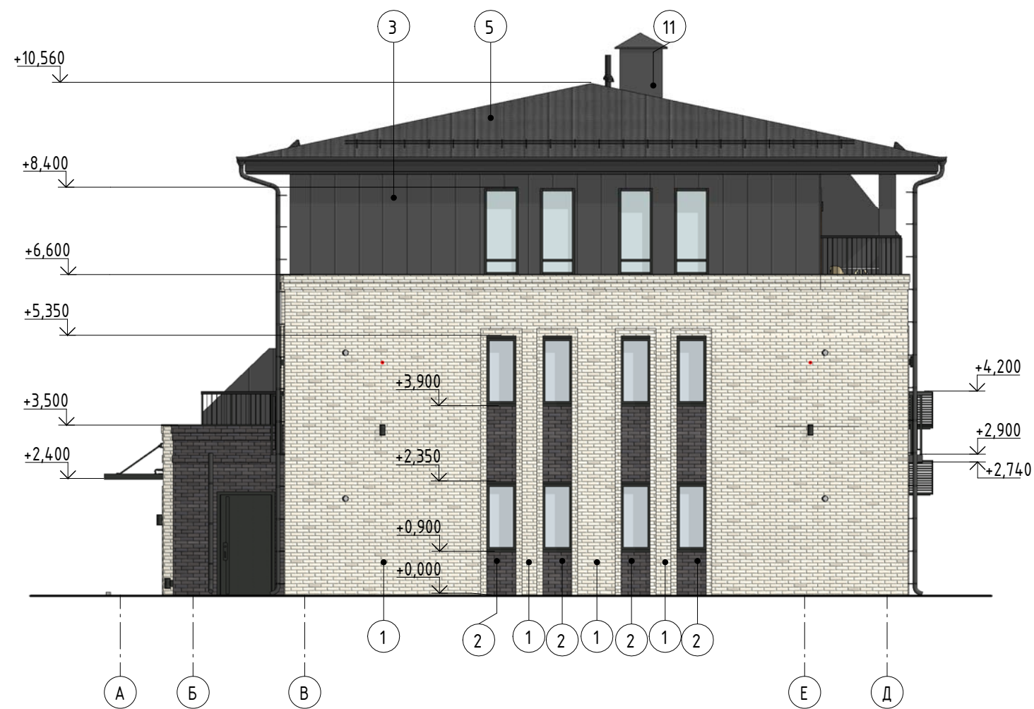
Фасад А-Д
