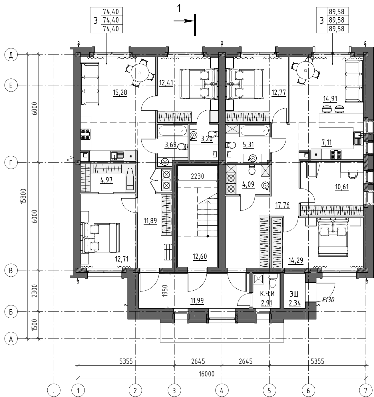
План этажа на отм. 0,000
