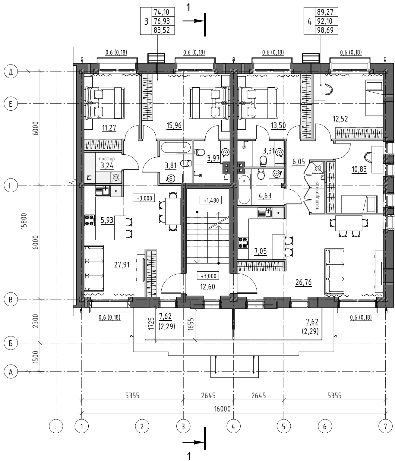
План этажа на отм. +3,000
